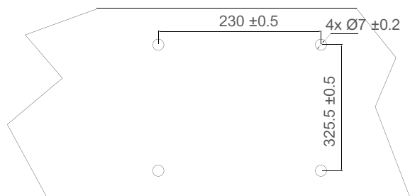
Backplane
